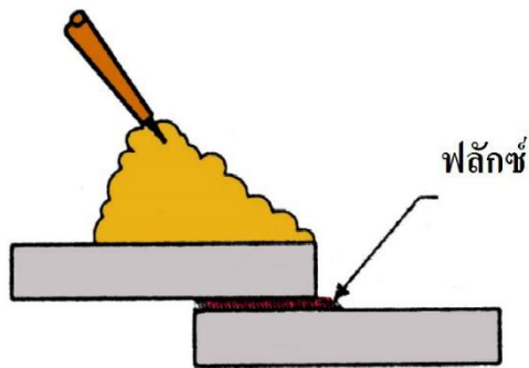
รูปที่ ๓.๙ แสดงการทำงานของฟลักซ์
