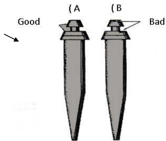
รูปที่ ๑.๕๙ แสดงภาพของหัวฉีดตัดแก๊ส (A) สภาพที่ดี (B) สภาพที่ชำรุด
