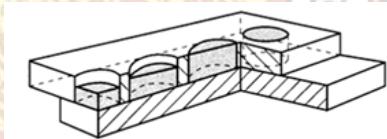
(ฑ) รอยเชื่อมรู (Plug Weld)
