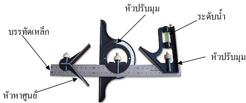
รูปที่ 6.12 แสดงลักษณะจากเหล็กเครื่องมือขนาดความยาว 24 นิ้ว (60 ซม.)
