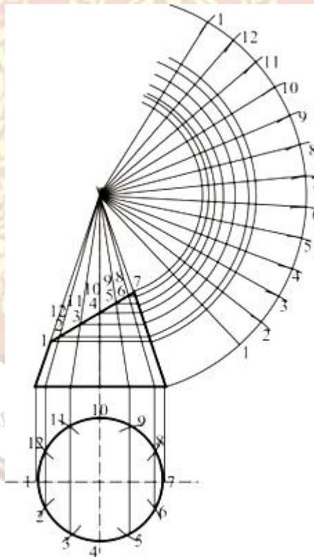
รูปที่ ๗.๑๔ แสดงเส้นฉายมายังแผ่นคลี่
