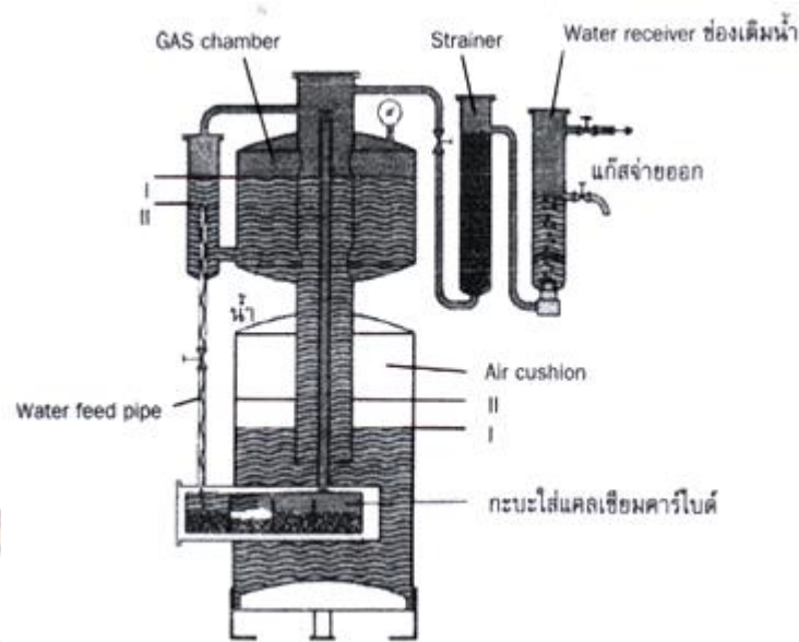
รูปที่ ๑.๕๗ แสดงเครื่องกำเนิดแก๊สอะเซทิลีนแบบเติมน้ำลงในแคลเซียมคาร์ไบด์ ที่มา : สมบูรณ์ เต็งหงษ์เจริญ. ม.ป.ป. : ๒๕
