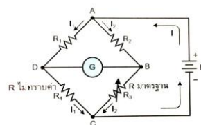
วงจรบริดจ์วีตสโตน
