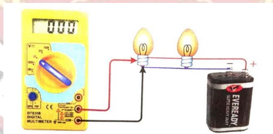
รูปที่ 9.6 การต่อดิจิตอลมัลติมิเตอร์วัดแรงดันไฟฟ้ากระแสตรง
