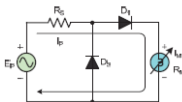
(ก) จ่ายไบแอสตรงให้ D_1
