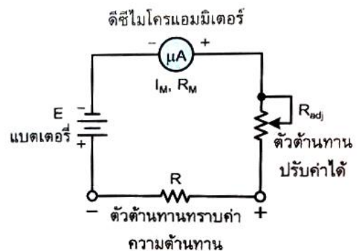
(ข) วงจร
