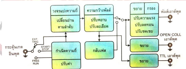
บล็อกไดอะแกรมเครื่องกำเนิดสัญญาณพัลส์
