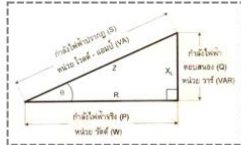
กำลังไฟฟ้าตอบสนองเกิดกับอุปกรณ์ตัวเหนี่ยวนำ (L)
