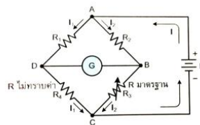
วงจรบริดจ์แบบสโตน
