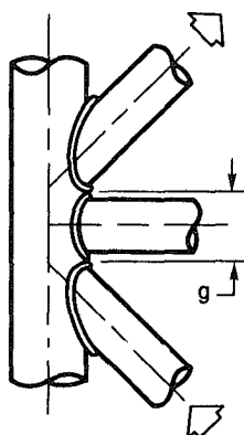
① K(T-K)
