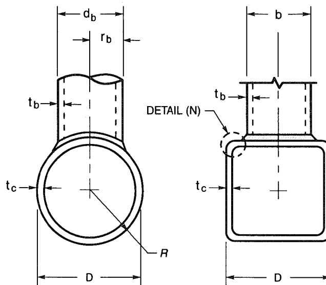
(M) GEOMETRIC PARAMETERS
