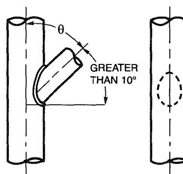
(D) Y-CONNECTION
