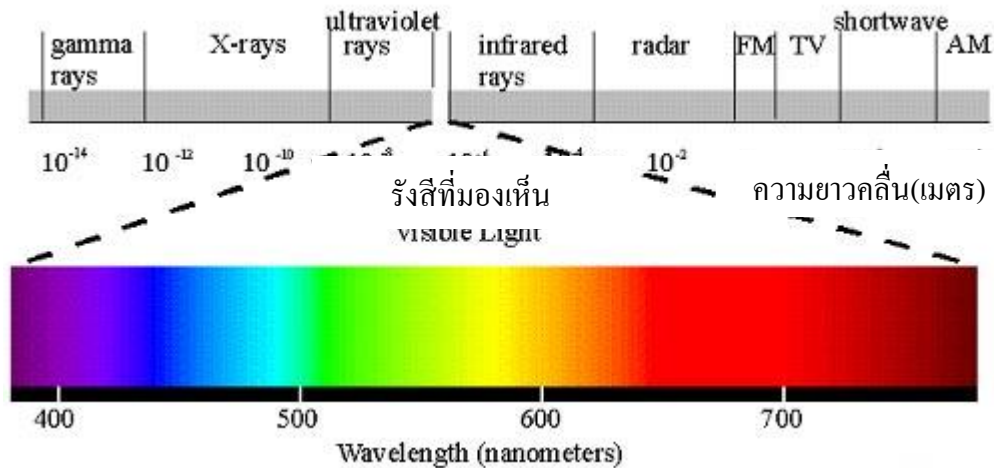
รูปที่ ๗ สเปกตรัมของคลื่นแม่เหล็กไฟฟ้า
