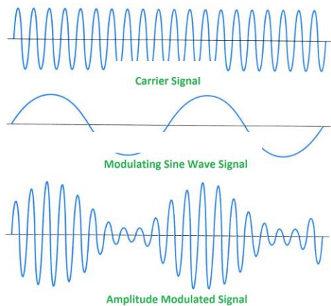
รูปที่ ๘ การผสมสัญญาณระบบ AM
