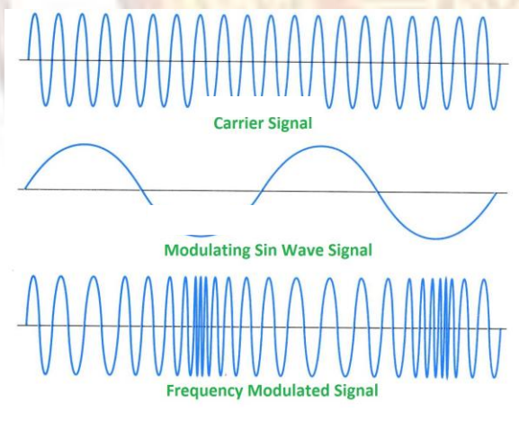
รูปที่ ๙ การผสมสัญญาณระบบ FM
