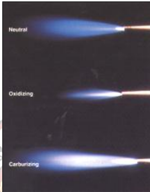
รูปที่ 3.14 แสดงเปลวแก๊สอะเซทิลีนกับออกซิเจน ในการเล่นประสาน
