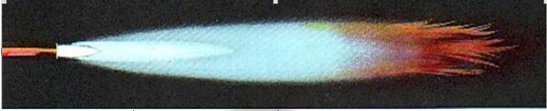
รูปที่ 1.46 แสดงเปลวคาร์บูไรซิง (Carburizing Flame)
