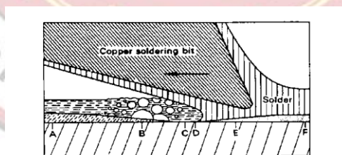
รูปที่ 9.7 แสดงปฏิกิริยาของฟลักซ์ขณะทำการบัดกรี
