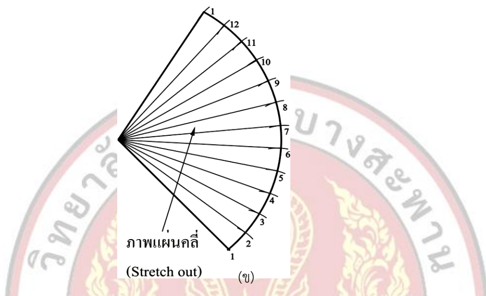
รูปที่ 7.9 แสดงเส้นต่าง ๆ ของการเขียนแบบแผ่นคลี่ด้วยวิธีเส้นรัศมี ที่มา : สุชาติ กิจพิทักษ์, 2540 : 154
