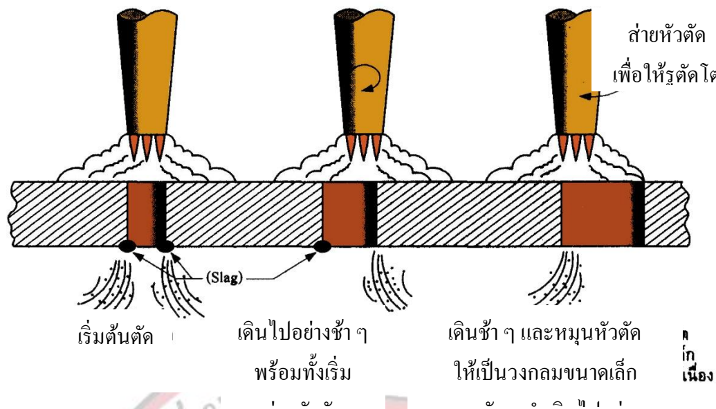
รูปที่ 4.15 แสดงการสายหัวตัดให้เป็นรูปวงกลมขนาดเล็กสำหรับการตัดเหล็กหนา
