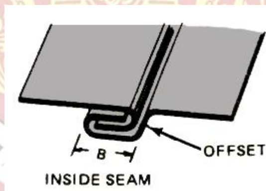
รูปที่ 8.6 แสดงการล็อกย่ำตะเข็บด้านใน(Inside seam)
