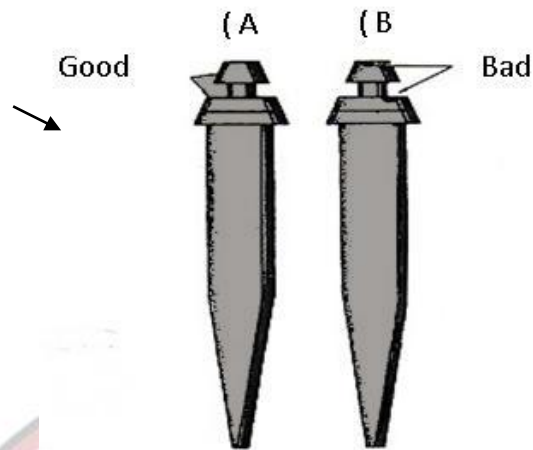
รูปที่ 1.59 แสดงบ่าของหัวฉีดตัดแก๊ส (A) สภาพที่ดี (B) สภาพที่ชำรุด
