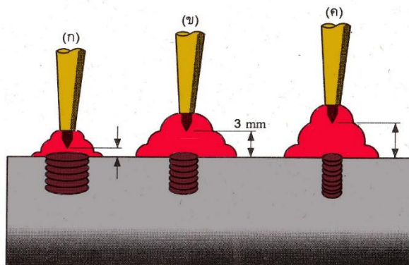
รูปที่ 1.54 แสดงระยะห่างระหว่างปลายของกรวยไฟกับผิวหน้าของงาน
