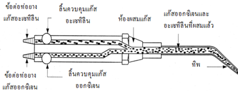
รูปที่ 1.40 แสดงลักษณะภายในของหัวเชื่อม ที่มา : นริศ ศรีเมฆ,พิชัย โอภาสอนันต์. 2543 : 41
