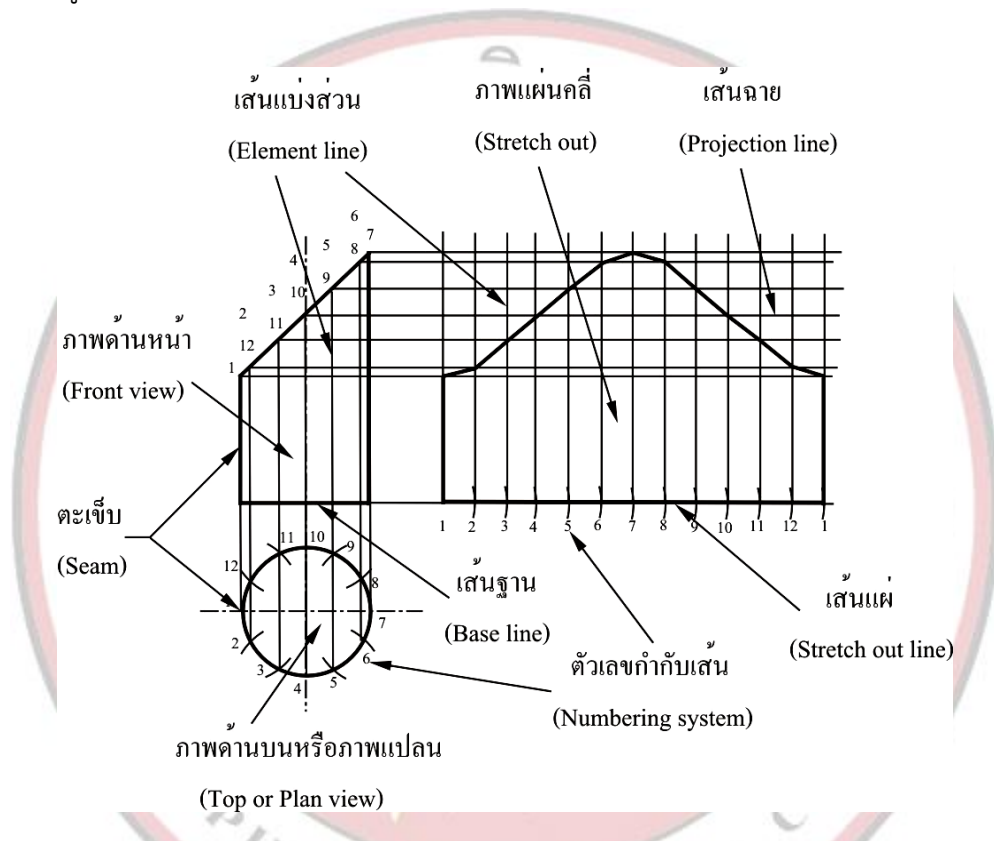
รูปที่ 7.4 แสดงความหมายของเส้นในแบบแผ่นคลี่
