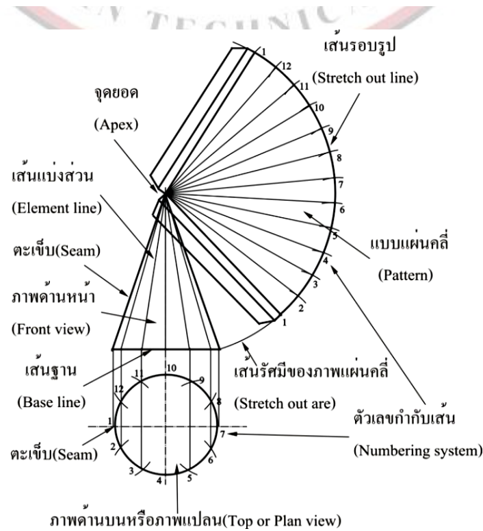
รูปที่ 7.8 แสดงงานผลิตภัณฑ์ที่ใช้หลักการเขียนแบบแผ่นคลี่ด้วยวิธีเส้นรัศมี
