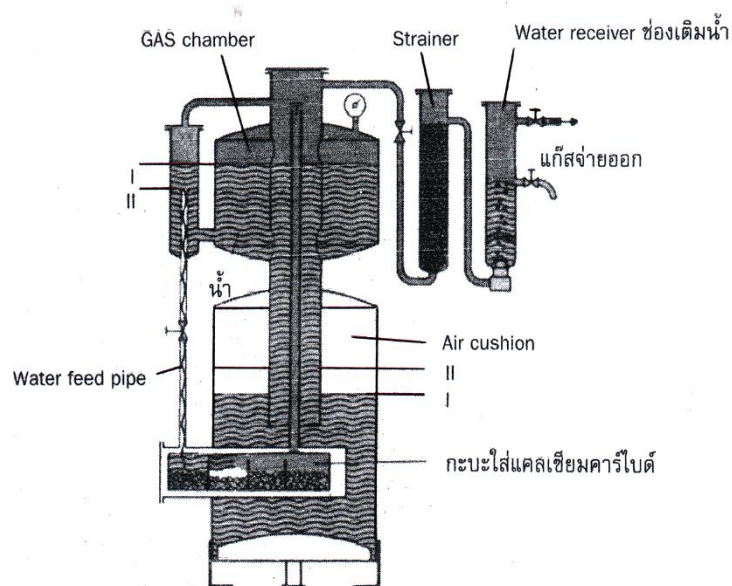
รูปที่ 1.57 แสดงเครื่องกำเนิดแก๊สอะเซทิลีนแบบเติมน้ำลงในแคลเซียมคาร์ไบด์
