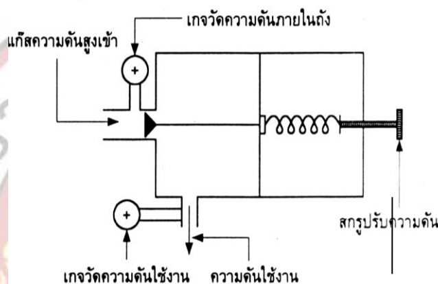
รูปที่ 1.34 แสดงลักษณะหลักการทำงานของหัวปรับความดันแบบขั้นเดียว
