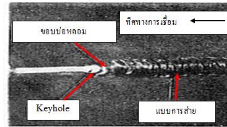
รูปที่ 1.50 แสดงการเชื่อมที่ทำให้เกิดรูกุญแจ (Keyhole)
