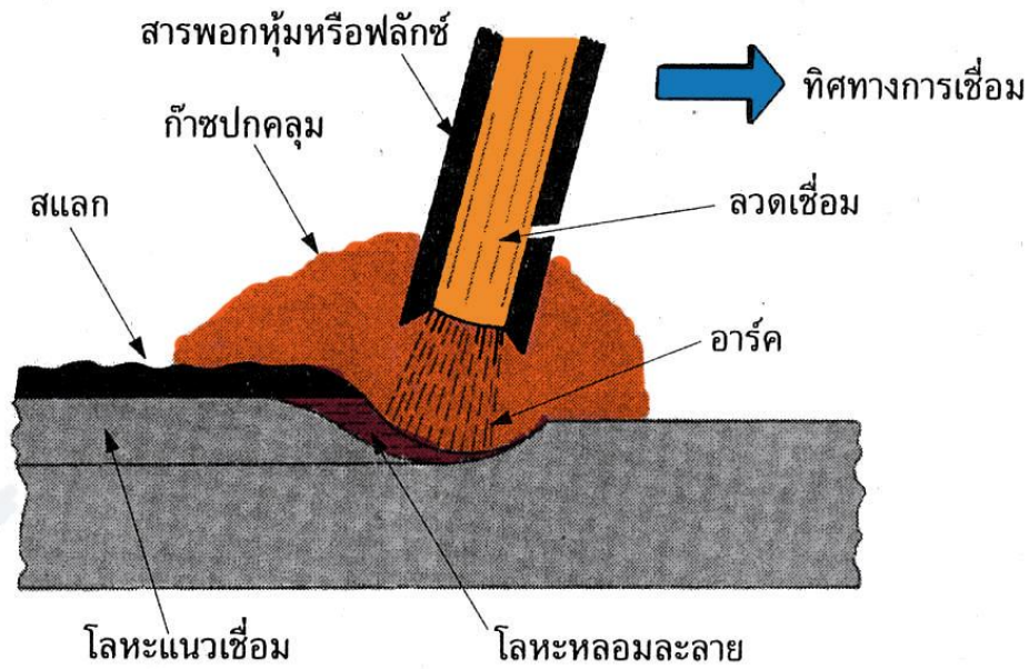
รูปที่ 5.1 แสดงองค์ประกอบของการเชื่อมอาร์กลวดหุ้มฟลักซ์
