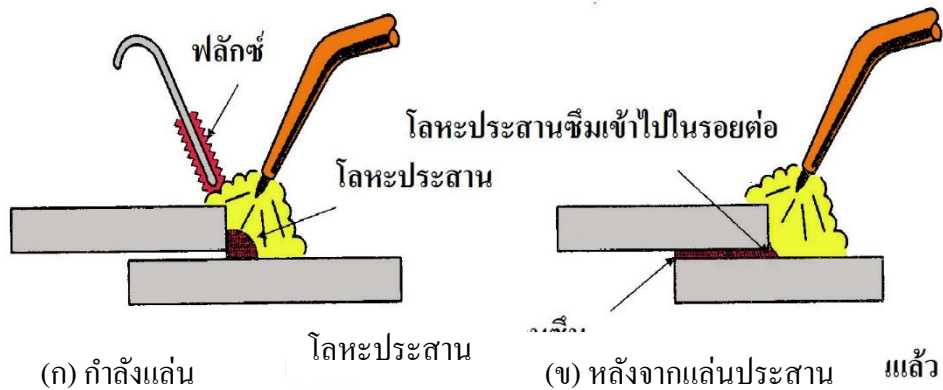
รูปที่ 3.3 แสดงรูปการซึมผ่านการเล่นประสาน
