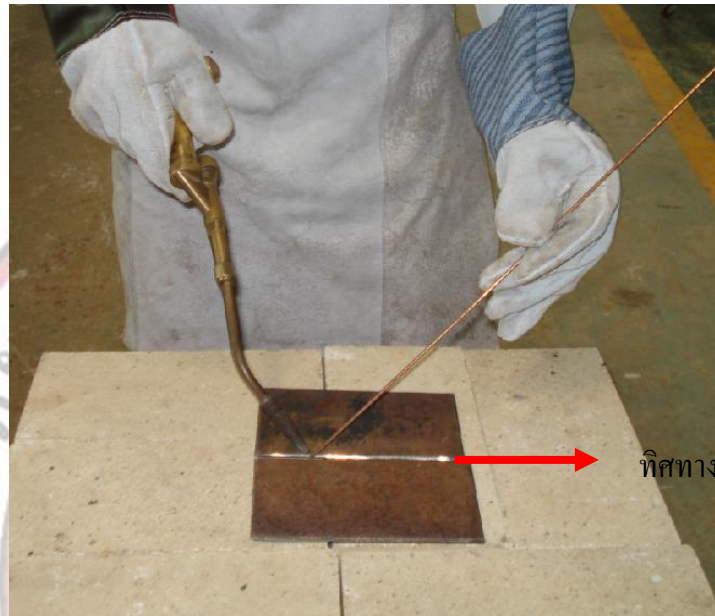
รูปที่ 1.49 แสดงตำแหน่งหัวเชื่อมและลวดเชื่อมสำหรับการเชื่อม Forehand Welding
