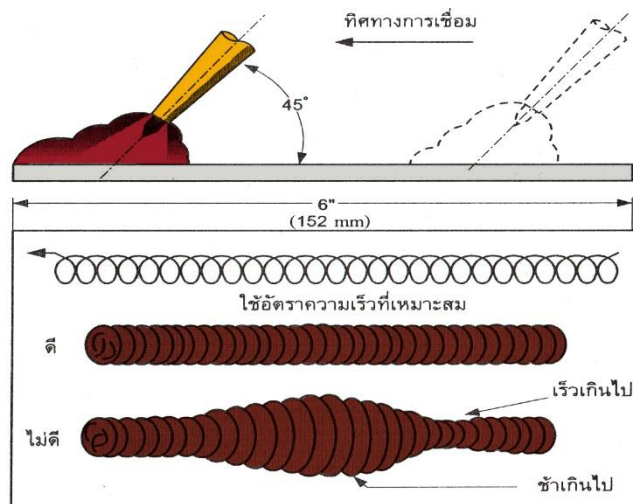
รูปที่ 1.52 แสดงผลที่เกิดจากการใช้อัตราความเร็วในการเคลื่อนหัวทิวที่แตกต่างกัน
