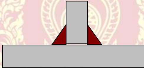
รูปที่ 5.66 แสดงการเชื่อมต่อนี้ที่แบบเชื่อมสองด้าน
