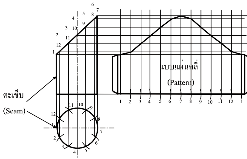
รูปที่ 7.5 แสดงแบบแผ่นดักที่เพื่ตะเข็บ
