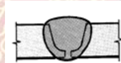
(ฉ) รอยเชื่อมชนรูป U ด้านเดียว
