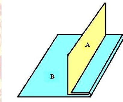
รูปที่ 8.9 แสดงลักษณะของตะเข็บพับชั้นเดียว
