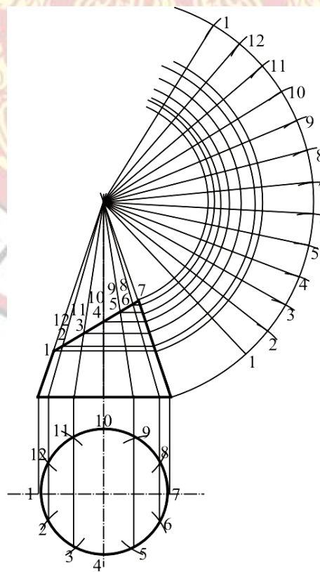
รูปที่ 7.14 แสดงเส้นฉายมายังแผ่นคลี่
