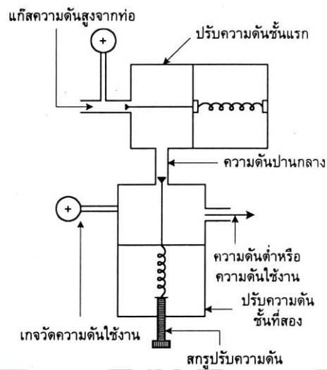
รูปที่ 1.31 แสดงลักษณะหลักการทำงานของหัวปรับความดันแบบสองชั้น
