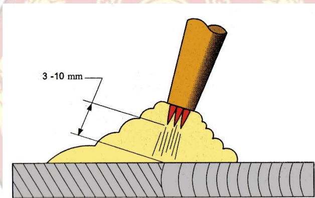
รูปที่ 4.9 แสดงระยะห่างระหว่างกรวยไฟกับชิ้นงานที่เหมาะสมในการตัด
