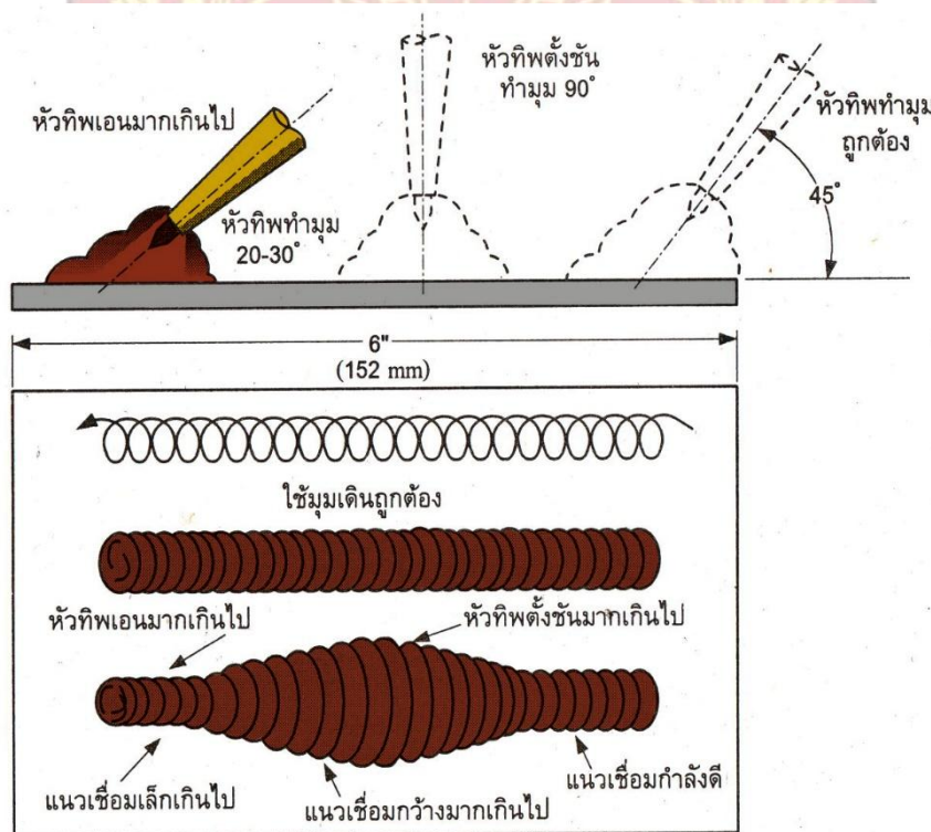
รูปที่ 1.53 แสดงลักษณะของแนวเชื่อมเมื่อมุมในการเชื่อมเปลี่ยนไป ขณะเคลื่อนหัวทิวไปข้างหน้า
