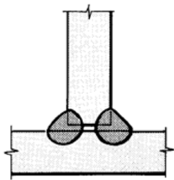
(ฎ) รอยเชื่อมฉากสองด้าน (Flare V Weld)
