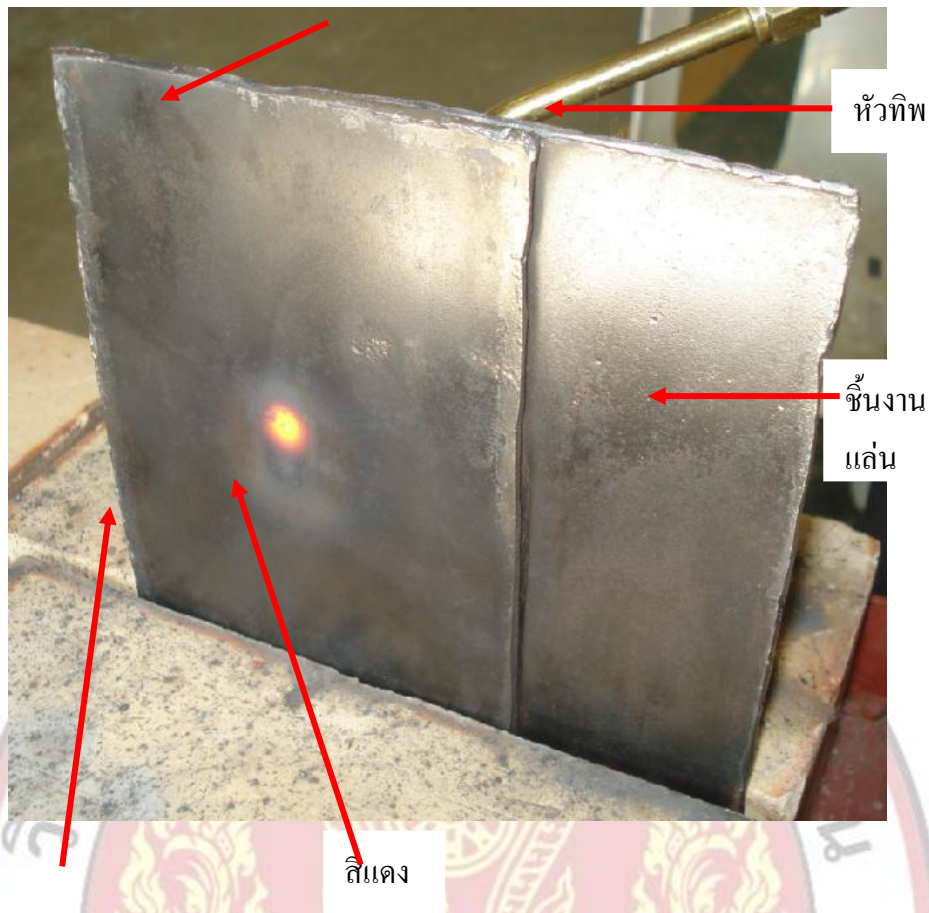
รูปที่ 3.18 แสดงความร้อนจากด้านหน้าที่เผาด้วยเปลวไฟจะส่งผ่านมายังชิ้นงานที่เกยอยู่ด้านหลังจนกระทั่งร้อนแดง
