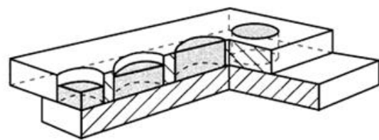
(ฑ) รอยเชื่อมอุด (Plug Weld)
