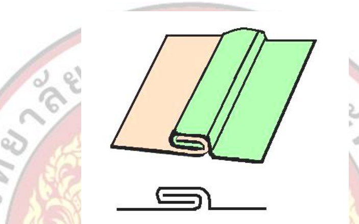
รูปที่ 8.5 แสดงการล็อกย่ำตะเข็บด้านนอก(Outside seam)
