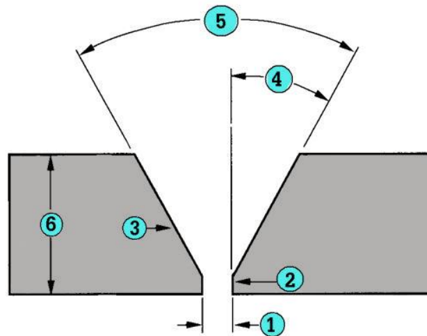
รูปที่ 2.4 แสดงรูปรอยเชื่อมบากร่อง ที่มา : อำนาจ ทองแสน, จริญญา พรหมสุทธิ 2546 : 36
