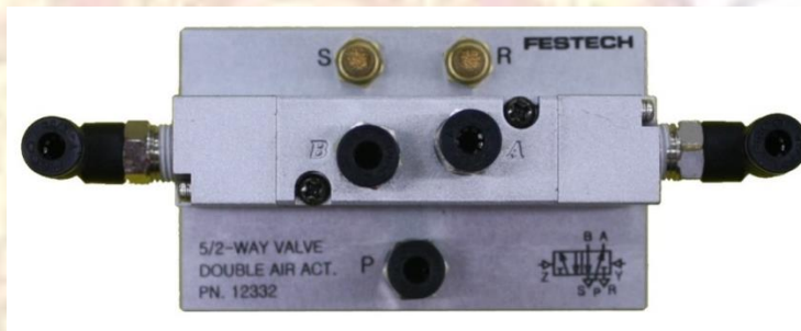
รูปแสดงโครงสร้างและสัญลักษณ์ของวาล์ว 5/2 แบบบังคับการทำงานด้วยลม
