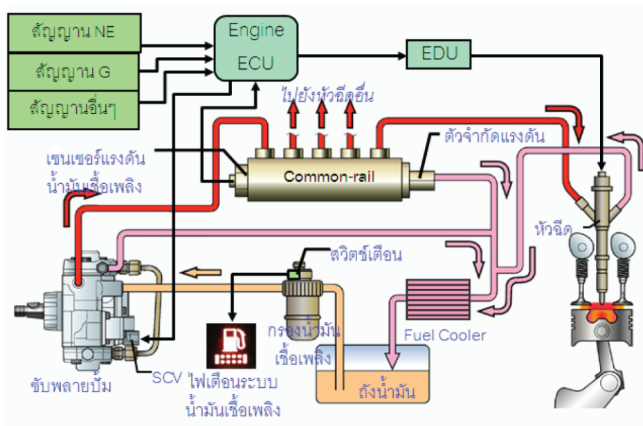
ภาพที่ 2.5 ส่วนประกอบของระบบคอมมอนเรล เครื่องยนต์ 1KD-FTV
