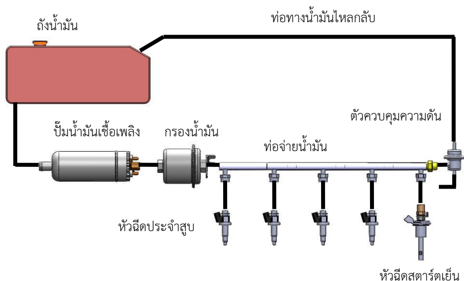
รูป ส่วนประกอบของระบบเชื้อเพลิง
