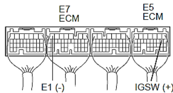
ภาพที่ 2.14 วัดแรงดันไฟฟ้าของขั้วต่อ ECM ระหว่างขั้ว IGSW – E1
