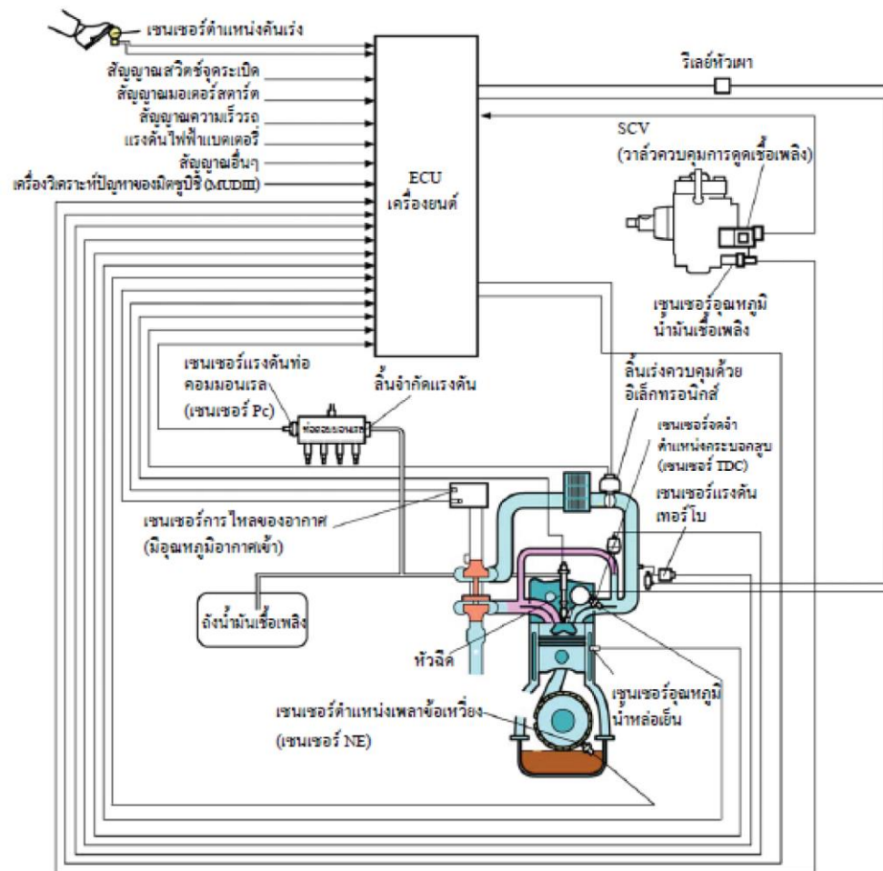
ภาพที่ 2.3 โครงสร้างของระบบคอมมอนเรล เครื่องยนต์ 4D-56
