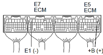
ภาพที่ 2.13 วัดแรงดันไฟฟ้าของขั้วต่อ ECM ระหว่างขั้ว +B – E1
