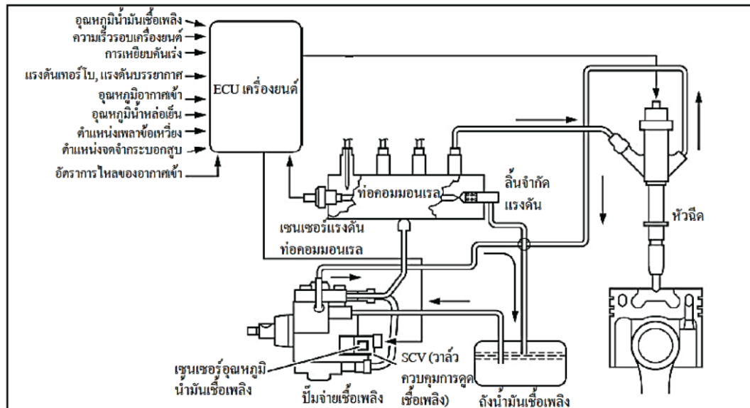
ภาพที่ 2.4 ส่วนประกอบของระบบคอมมอนเรล เครื่องยนต์ 4D-56
