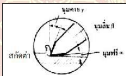
รูป แสดงลักษณะของคมสกัดทิศทางตัดแสดงผิวคายและมุม
