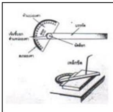
รูปที่ 3.4 แสดงลักษณะของบรรทัดวัดมุม และการใช้งาน
