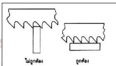
รูป แสดงการเลือกใช้ความหยาบ ความละเอียดของฟันเลื่อยให้เหมาะสมกับความหนาของชิ้นงาน
