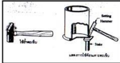
รูปที่ 2.5 แสดงลักษณะของค้อนยั่วตะเข็บ และการใช้งาน
